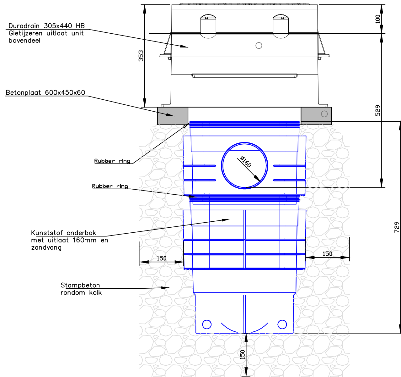
Vooraanzicht
