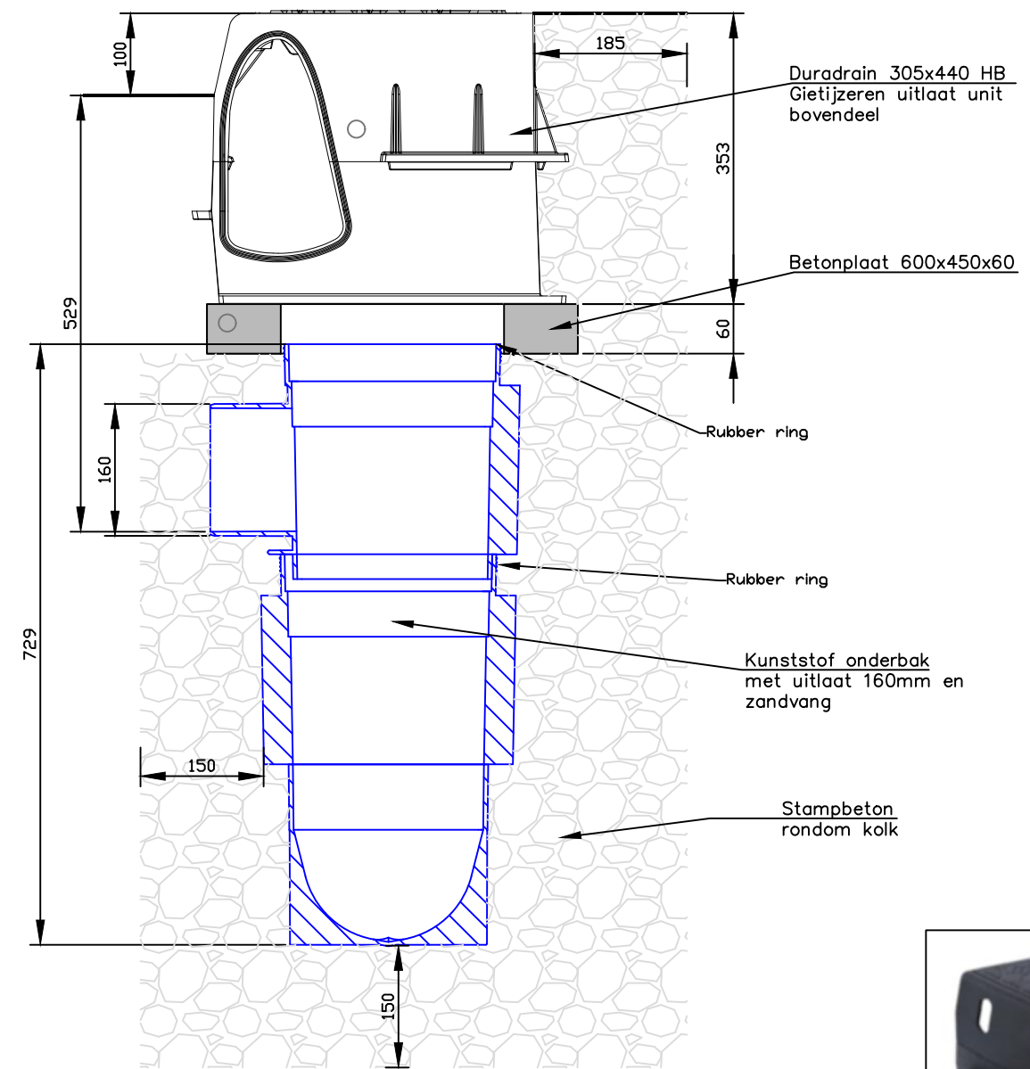
Zijaanzicht
